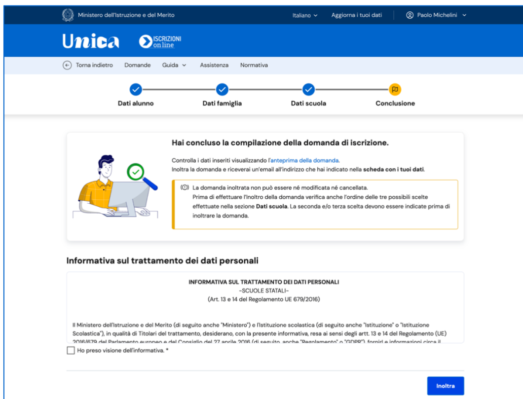
FIGURA 19 – SCHERMATA CONCLUSIONE
